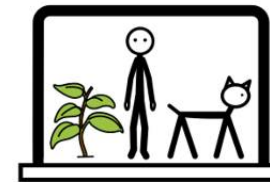
YMPÄRISTÖOPPI
