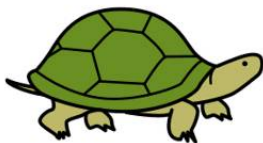
KILPIKONNA
