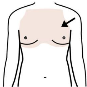
RINTAKEHÄ
