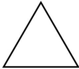
KOLMIO
