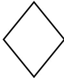
VINONELIÖ
