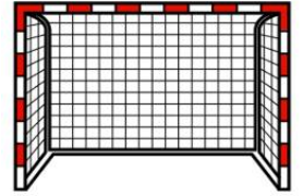
MAALI
